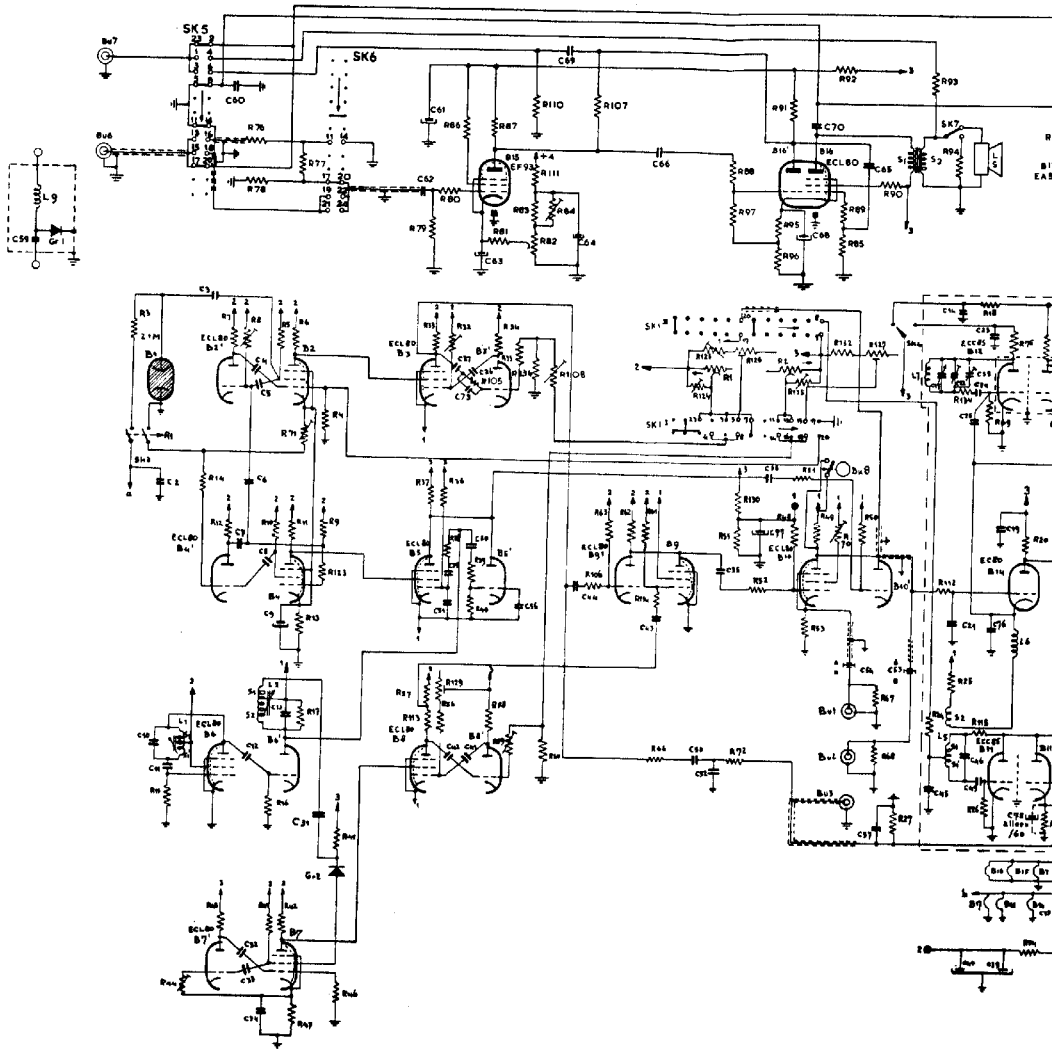
Fig. 19. Schema van de televisie-servicekoffer GM 2851/50 en GM 2851/60 (wijzigingen voorbehouden). Op verschillende plaatsen is de schakeling met de kast verbonden. De afregelweerstand R_{124} en R_{125} (bij SK_1 ) zijn vervallen. In sommige apparaten is aan R_{81} (aan katode van B_{15} ) een afregelweerstand R_{127} toegevoegd ( 180 \Omega - 1 ).
