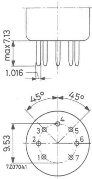
MINIATURE 7-PIN BASE (IEC 67-I-10a)
