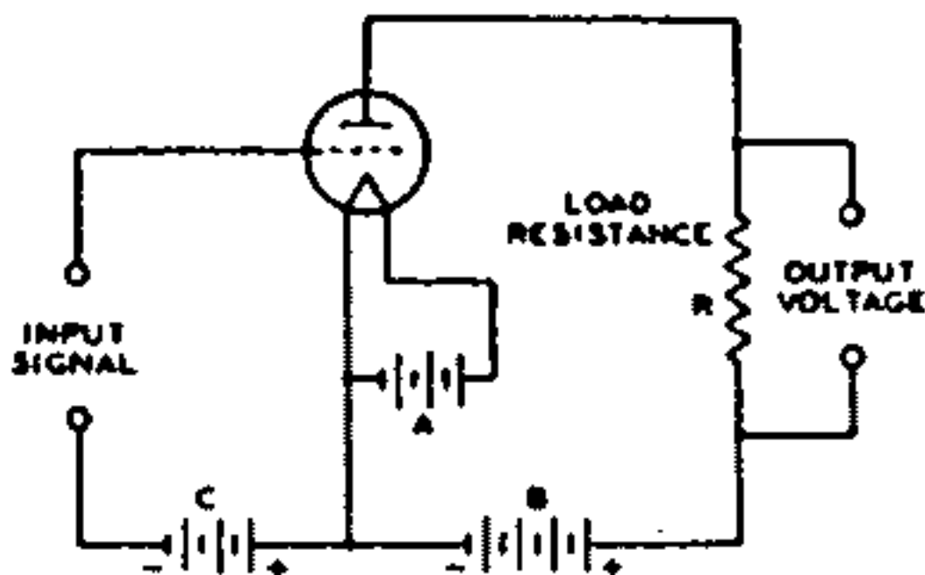
Fig. 35—Triode amplifier circuit.
