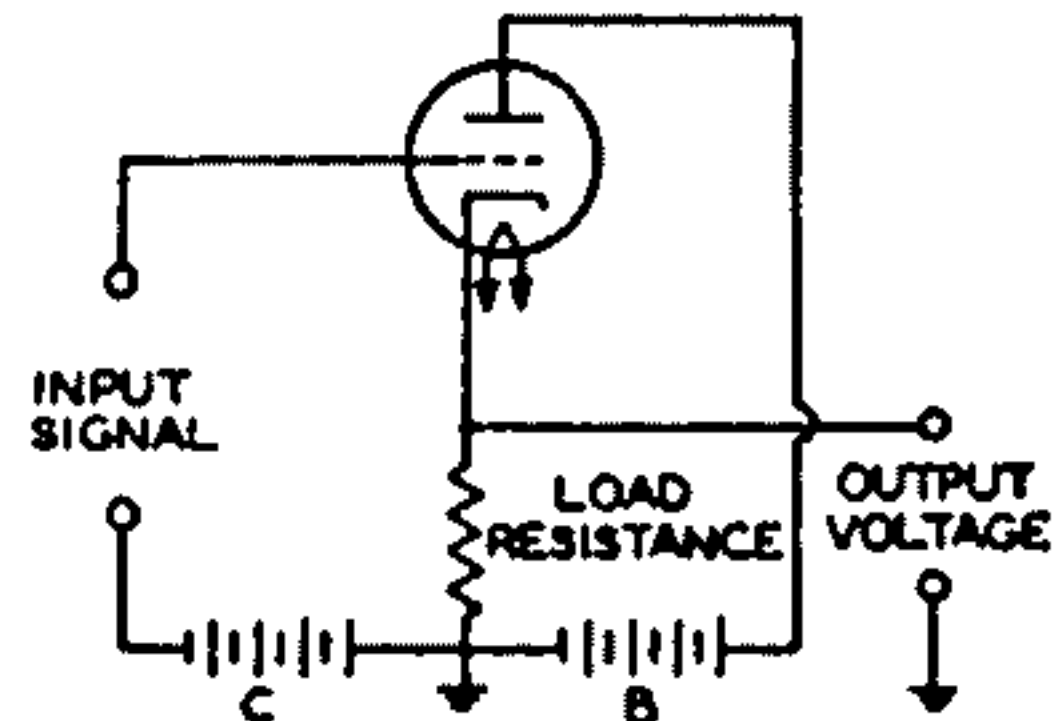
Fig. 51—Cathode-follower circuit.
