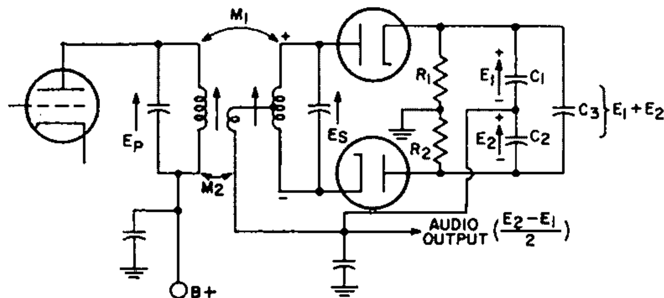
Fig. 33—Radio-detector circuit.
