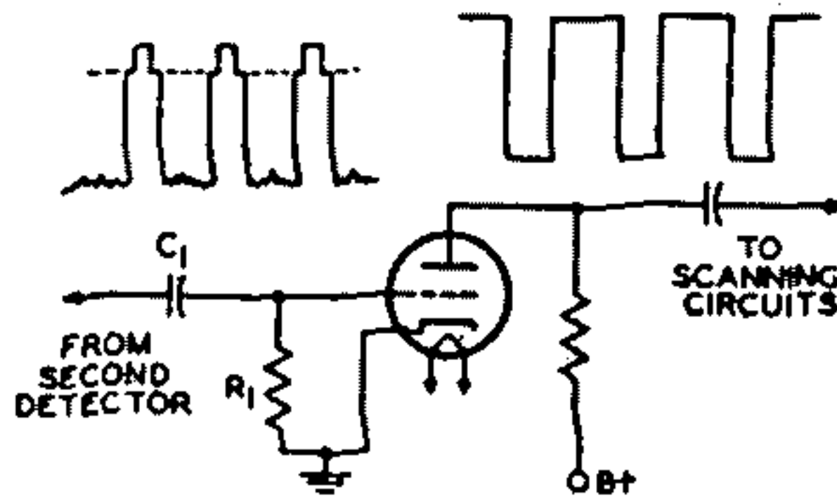
Fig. 80—Sync-separator circuit.
