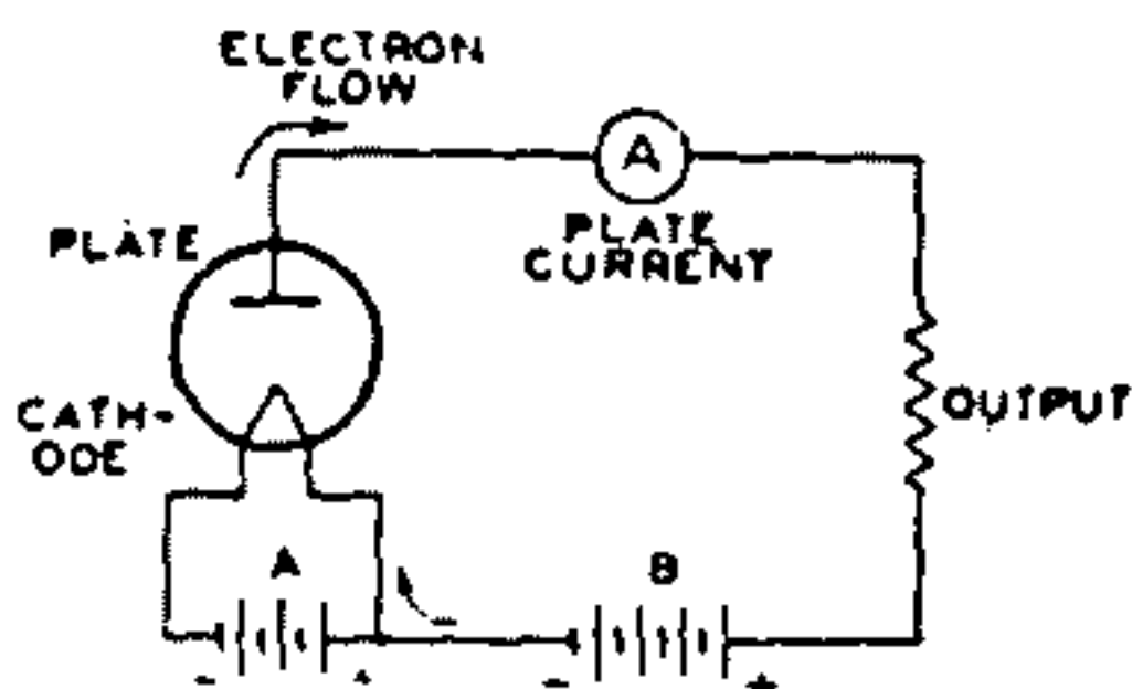
Fig. 3—Basic diode circuit.
