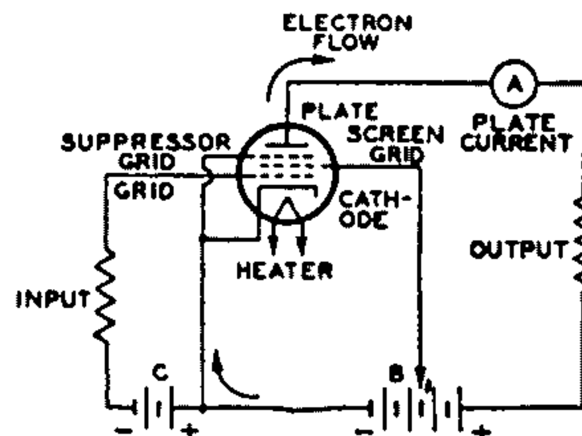
Fig. 8—Basic pentode circuit.
