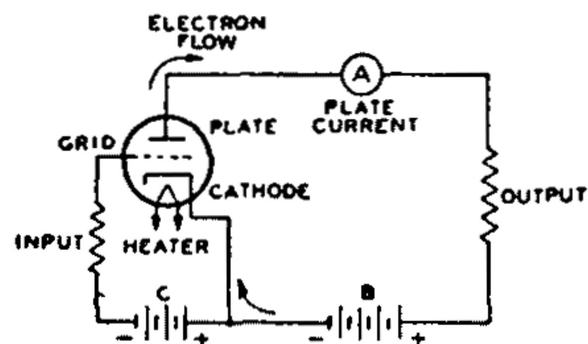
Fig. 6—Basic triode circuit.
