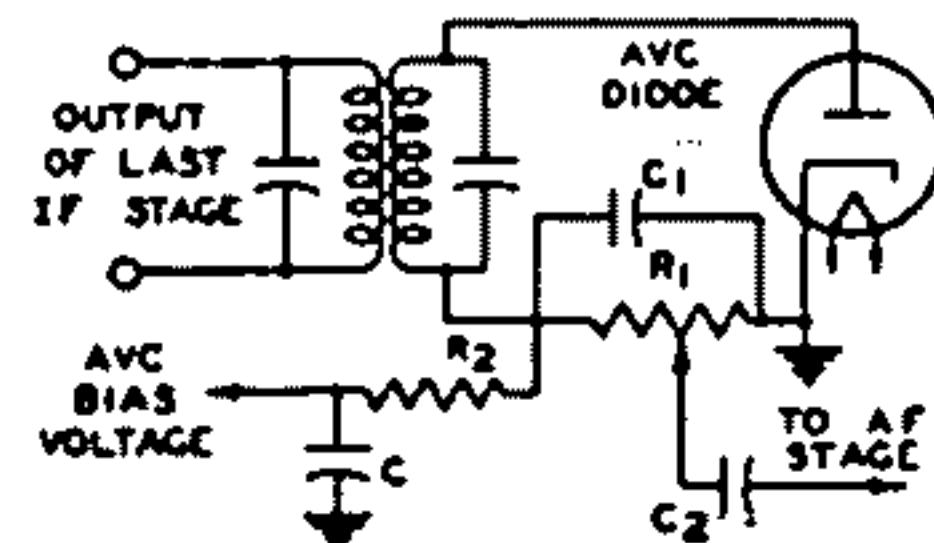
Fig. 61—Automatic-volume-control (avc) circuit.
