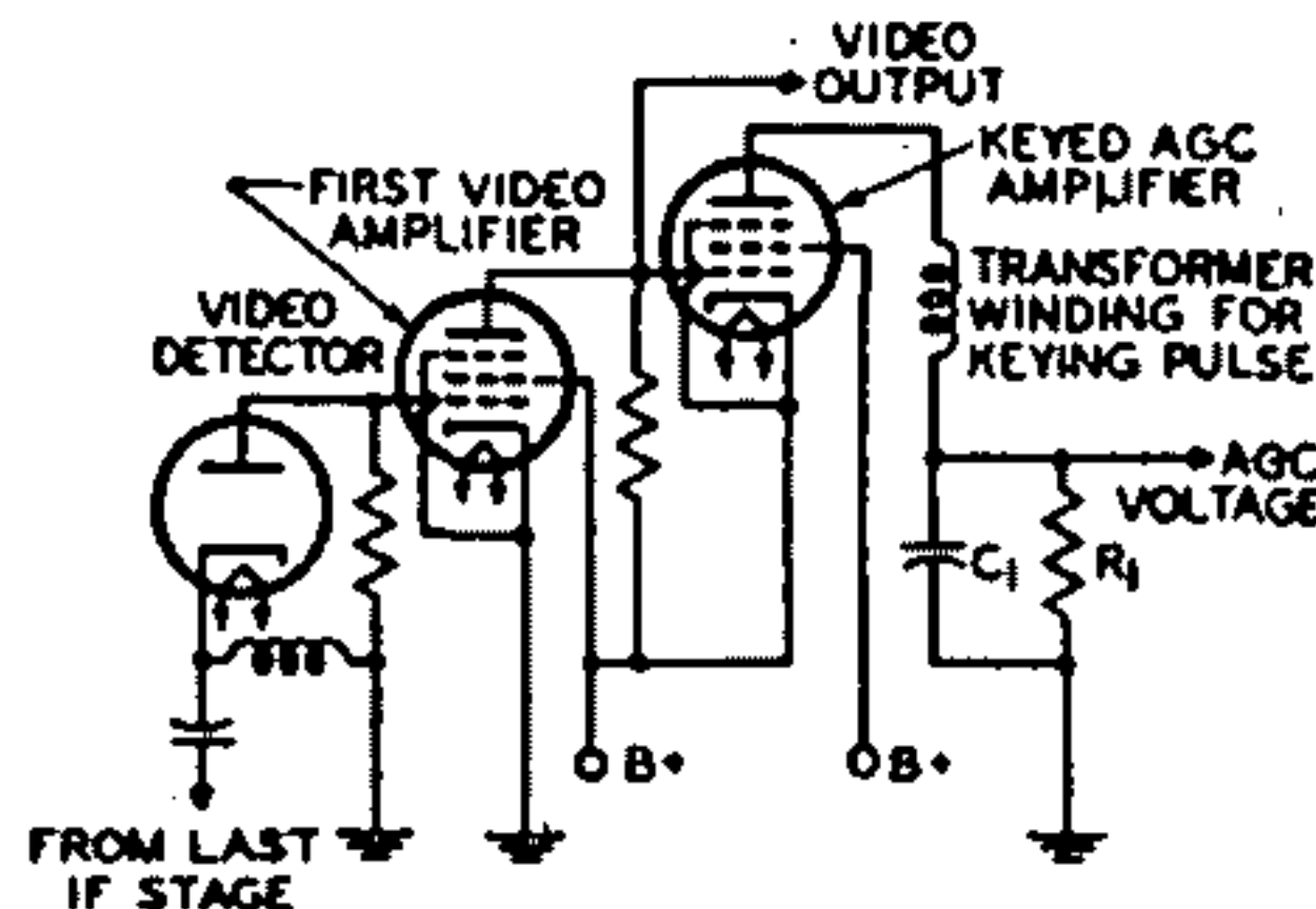
Fig. 64—"Keyed" agc circuit.
