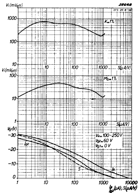
Abb. 7 Für eine Schirmgitterspannung von 60 V: Obere Kurve: Effektive Gitterwechselspannung als Funktion der Steilheit für 1% Quermodulation. Mittlere Kurve: Effektive Gitterwechselspannung als Funktion der Steilheit für 1% Modulationsbrümmen. Untere Kurven: Steilheit S und Anodenstrom I_a als Funktion der Spannung des ersten Gitters.
