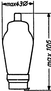
Kolbenabmessungen
